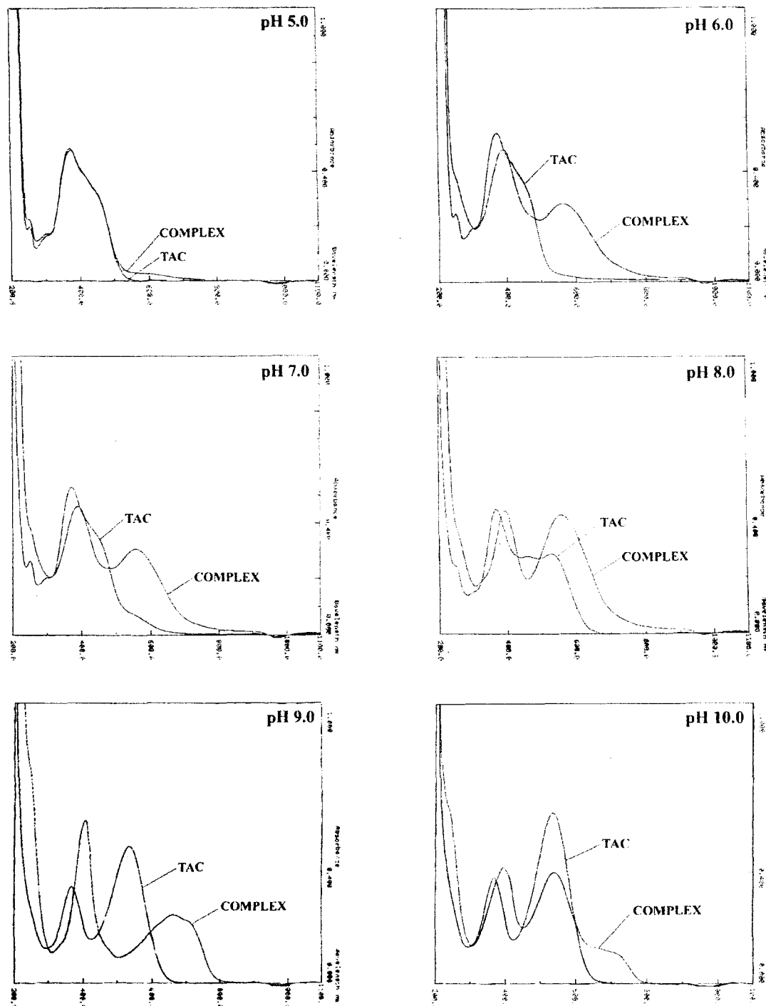
รูปที่ 3 แสดง UV-Vis spectra ของ TAC และสารประกอบเชิงซ้อนระหว่าง \text{Co}^{2+} กับ TAC ที่ pH 5-10
